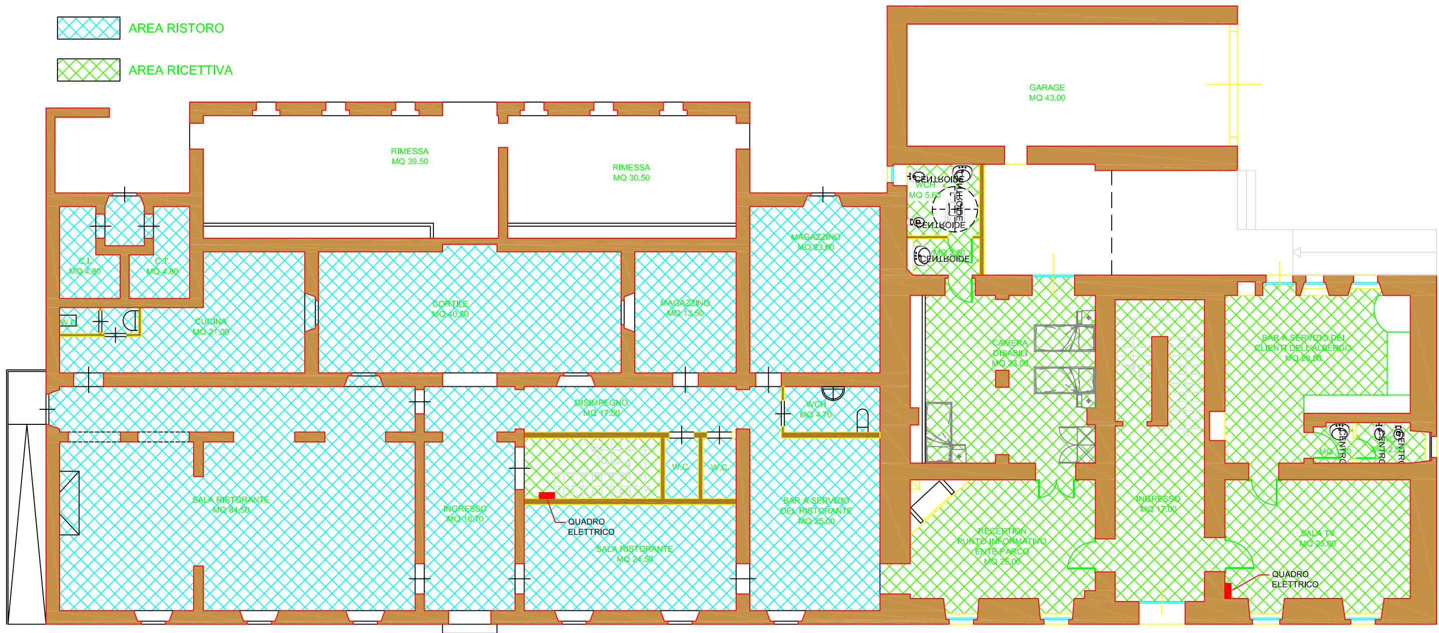
SOLUZIONE 2 – PALADINI DI CROGNALETO PIANTA PIANO TERRA IPOTESI DI PROGETTO
